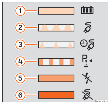
Abb. 230 Auf der Innenseite der Batterieladeklappe: Aufkleber mit Informationen zur Ladevorgangsanzeige.
