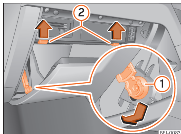
Abb. 50 Handschuhfach (Rechtslenker): Zugang zum Sicherungskasten.
