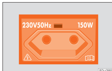
Abb. 146 Im Gepäckraum links: 230-Volt-Steckdose.
