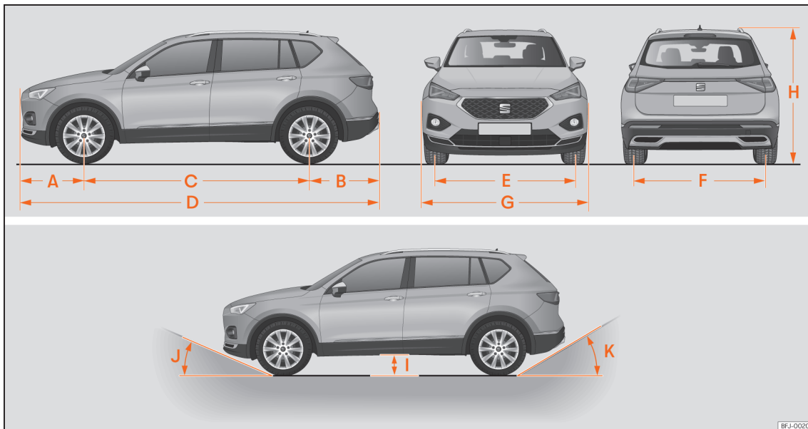
Abb. 259 Abmessungen
