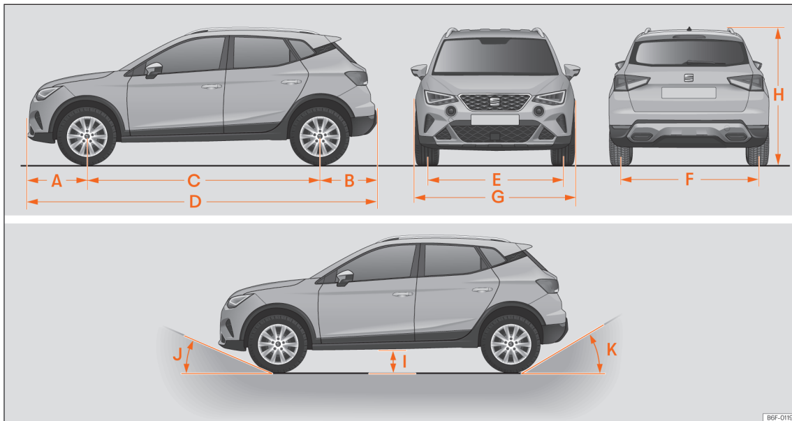
Abb. 203 Abmessungen und Winkel.
