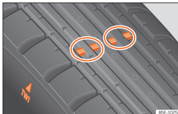
Abb. 188 Reifenprofil: Verschleißanzeiger.
