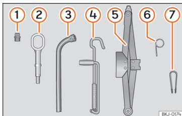
Abb. 156 Im Gepäckraum unter dem Gepäckraumboden: Bordwerkzeug.
