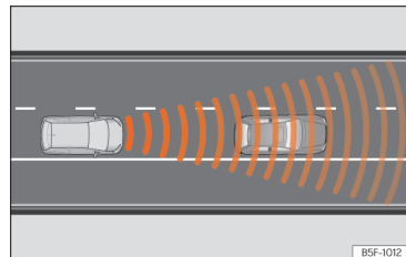
Abb. 95 Erkennungsbereich.
