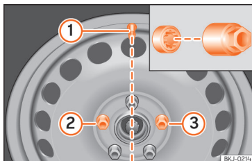
Abb. 195 Radwechsel: Reifenventil ① und Einbauort der Anti-Diebstahl-Radschraube ② oder ③.
