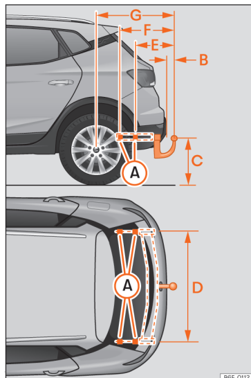
Abb. 151 Maße und Befestigungspunkte für den nachträglichen Einbau einer Anhängervorrichtung
