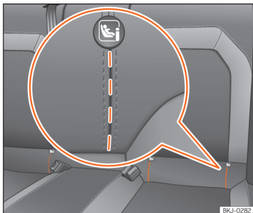
Abb. 37 Rücksitze: eingepprägte Schlitze für Zugriff auf die ISOFIX/i-Size-Halteösen.
