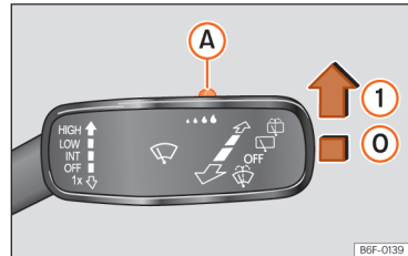
Abb. 77 Scheibenwischerhebel: Regensensor (A) einstellen.
