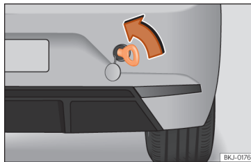
Abb. 157 Auf der rechten Seite des hinteren Stoßfängers: Eingeschraubte Abschleppöse.
