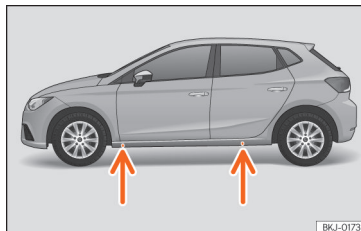
Abb. 189 Aufnahmepunkte für den Wagenheber.
