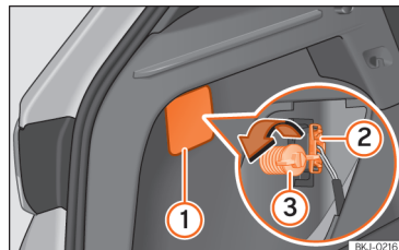
Abb. 161 Gepäckraum: Zugang zur Befestigungsschraube der Heckleuchte
