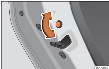
Abb. 56 Kindersicherung in der linken Tür
