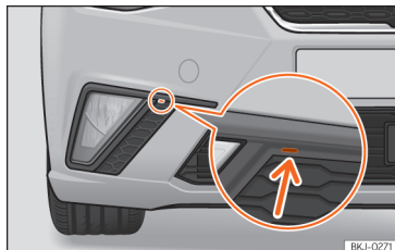
Abb. 163 Nebelscheinwerfer: Gitter abnehmen
