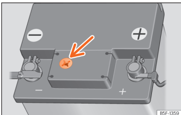
Abb. 178 Sichtfenster an der Oberseite der 12-Volt-Fahrzeugbatterie (Prinzipdarstellung).
