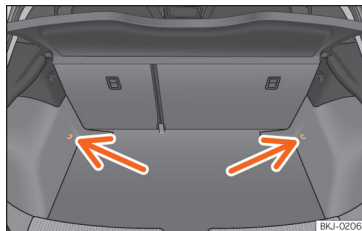
Abb. 140 Anordnung der Verzurrösen im Gepäckraum.
