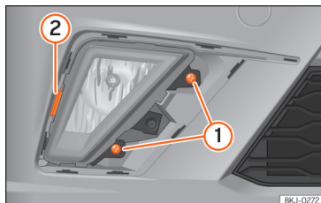
Abb. 164 Nebelscheinwerfer: Lampenträger ausbauen
