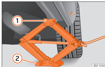
Abb. 190 Längsholm: Wagenheber ansetzen.
