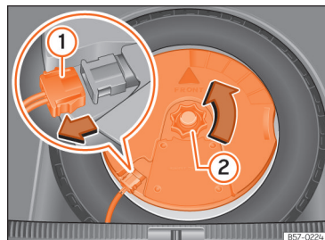
Abb. 182 Im Gepäckraum: Subwoofer ausbauen.
