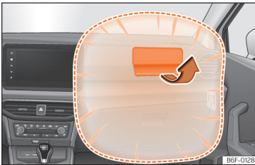
Abb. 29 Beifahrerairbag in der Instrumententafel
