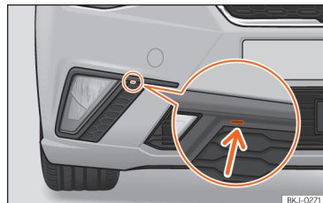
Abb. 164 Nebelscheinwerfer: Gitter abnehmen
