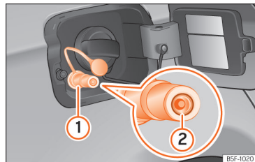
Abb. 147 Geöffnete Tankklappe: Gas-Einfüllstutzen ①, Dichttring des Einfüllstutzens ②.
