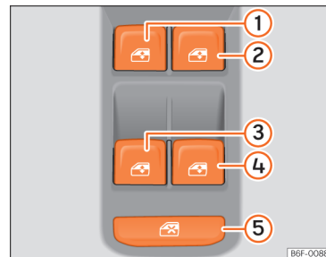
Abb. 84 Ausschnitt der Fahrertür: Tasten zum Bedienen der elektrischen Fensterheber
