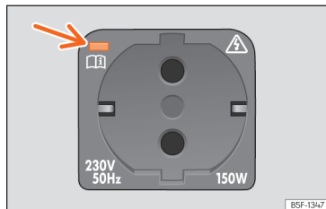
Abb. 163 Im Gepäckraum: 230-Volt-Steckdose.
