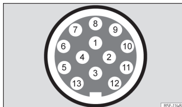
Abb. 196 Schematische Darstellung: Zuweisung der Steckverbinderstifte für Anhängerstrom.
