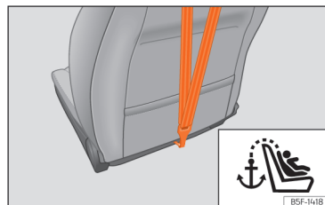
Abb. 50 Rückseite der Beifahrersitzlehne: Verankerung für den Top Tether Haltegurt.
