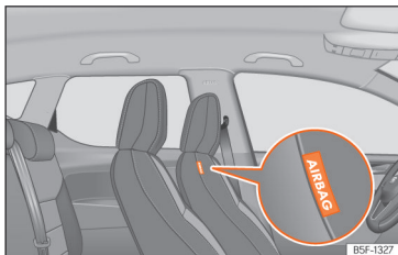
Abb. 34 Im Sitzlehnenpolster des Fahrersitzes: Center-Airbag.
