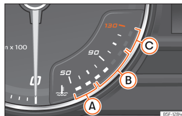
Abb. 10 Analoges Kombi-Instrument: Motorkühlmitteltemperatur-Anzeige.
