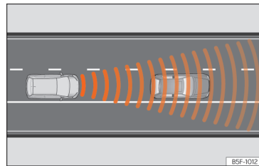
Abb. 123 Erkennungsbereich.
