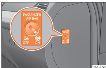
Abb. 32 Schlüsselschalter zum Ein- und Abschalten des Beifahrerairbags.
