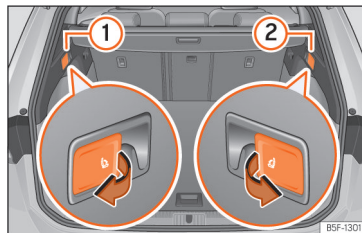
Abb. 100 Im Gepäckraum: Hebel zum Entriegeln der Rücksitzlehne.
