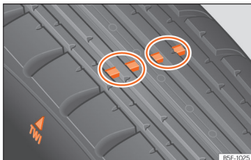
Abb. 233 Reifenprofil: Verschleißanzeiger.
