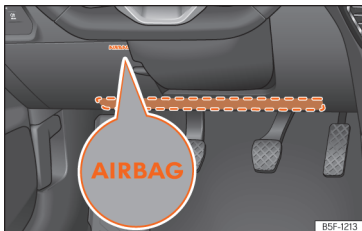
Abb. 39 Auf der Fahrerseite: Einbauort des Knieairbags.
