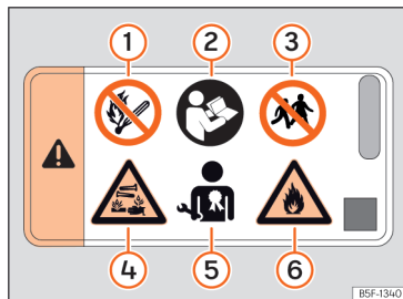
Abb. 231 48-Volt-Fahrzeugbatterie: Gefahrenwarnung
