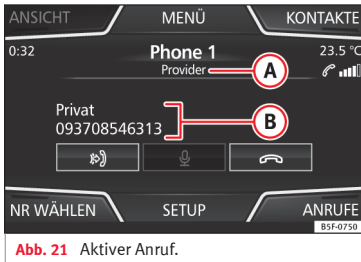
Abb. 21 Aktiver Anruf.
