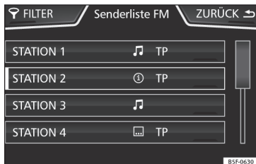
Abb. 9 Senderliste.
