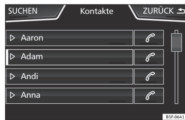
Abb. 24 Menü Kontakte.
