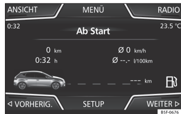
Abb. 31 Menü Reisedaten
